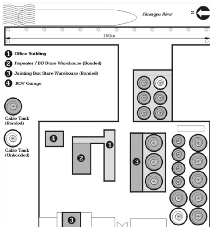
仓库总布置图
